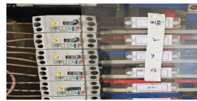
운정그린캠퍼스 옥외 전로 누전차단기 (양호)
