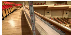
대강당 개방공간 추락 방지 난간 높이 (미흡)
